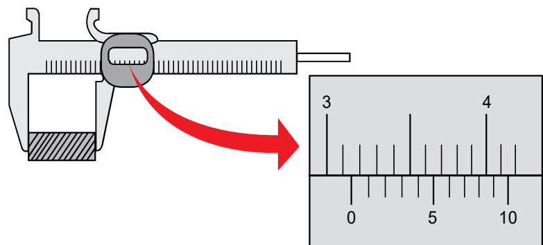
Gambar 5. Jangka sorong (pada gambar menunjukkan nilai 3,19cm)
